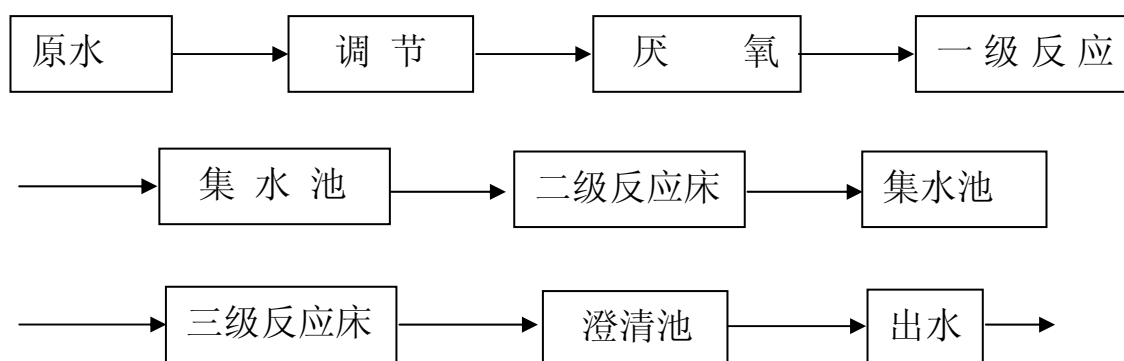
图8-1 典型矿化垃圾生物反应床流程
